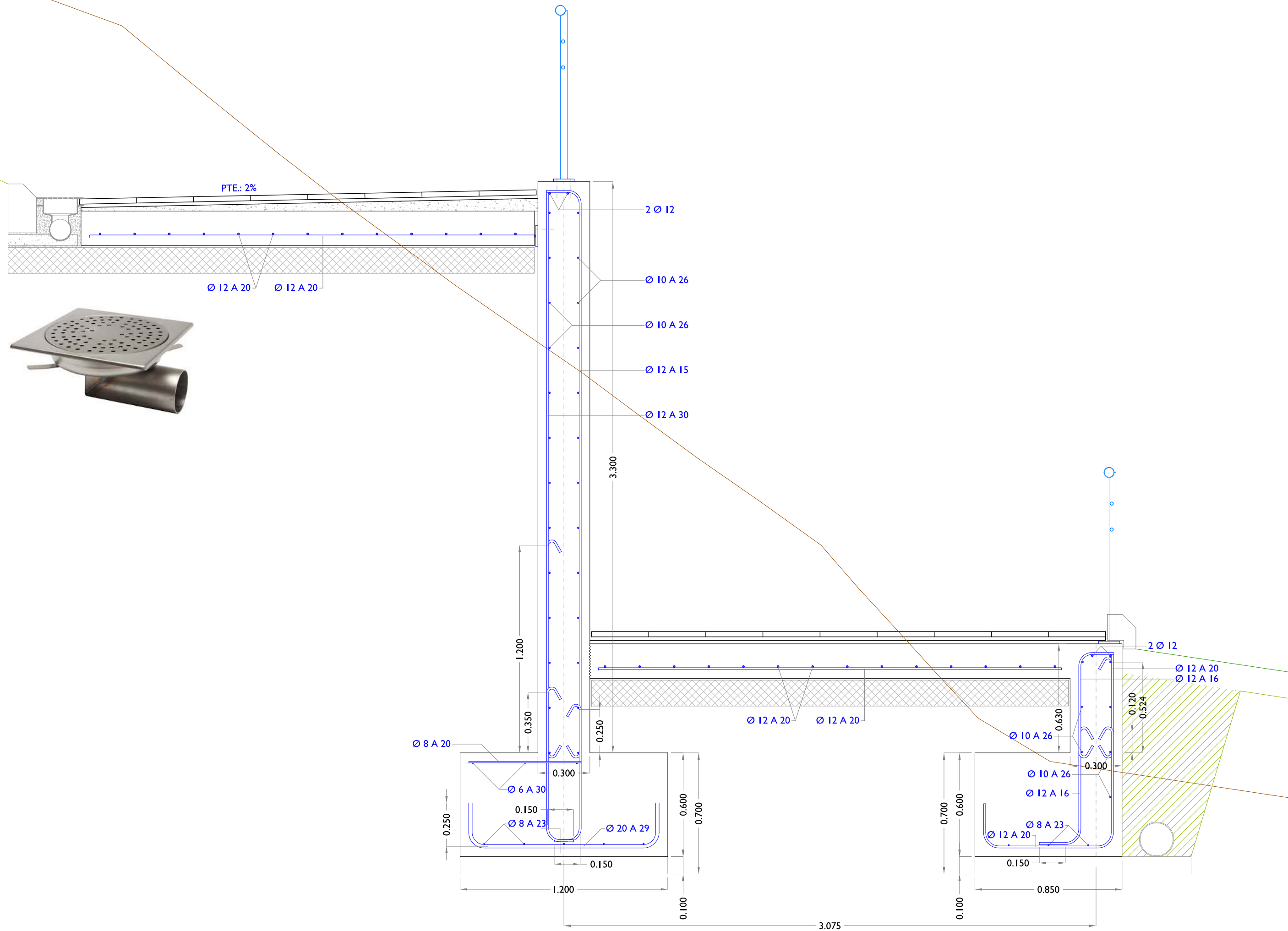
SECCIÓN GENERAL
